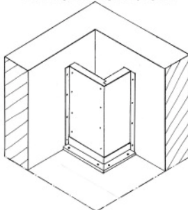
WAS 3-seitig, Kanal Direktmontage WAND (hier 2-seitiger Kanal) Senkrechte Montage
