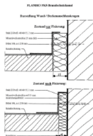
WAS Schnitt oberes Bild vor Montage unteres Bild nach Montage
